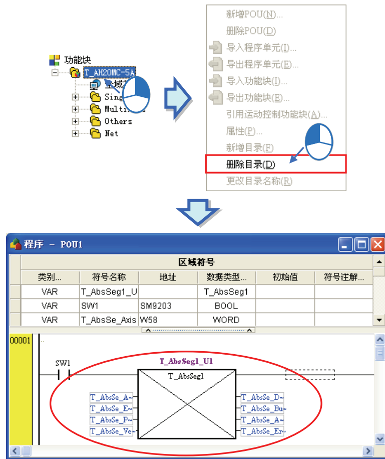
图 4 删除旧项目
